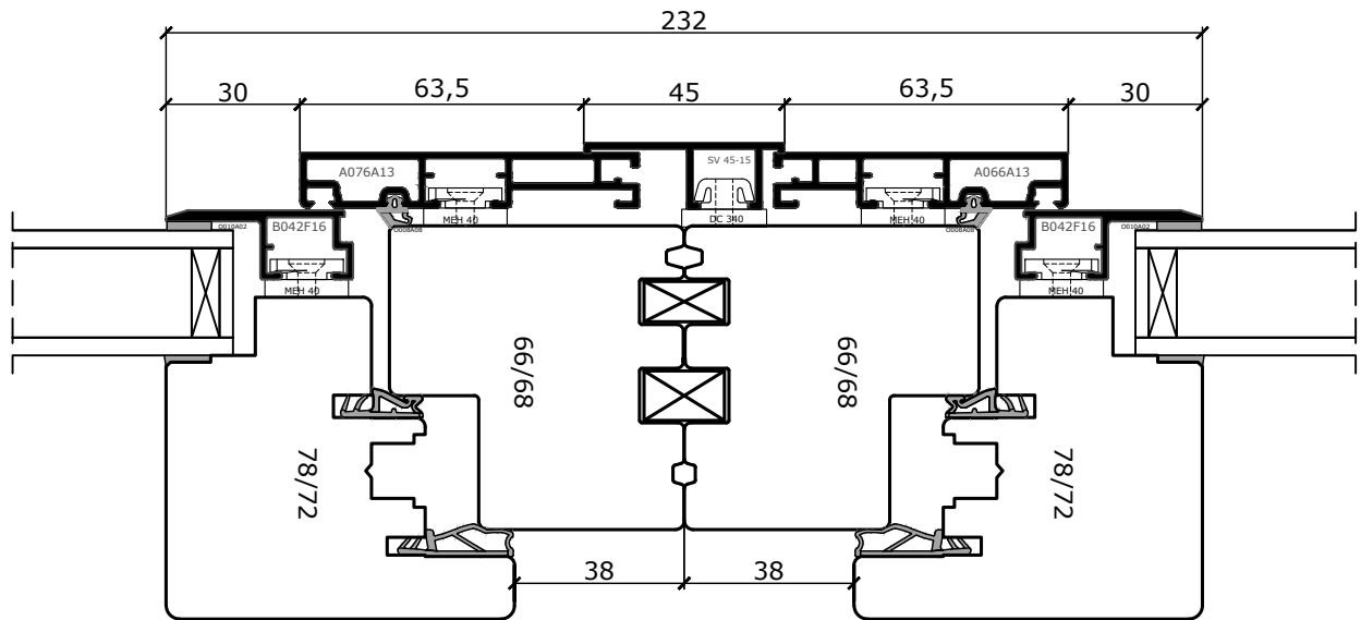
Verbreiterungsprofile
