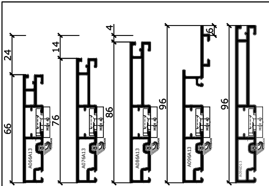
Ausführungsvarianten Blendrahmenprofil
