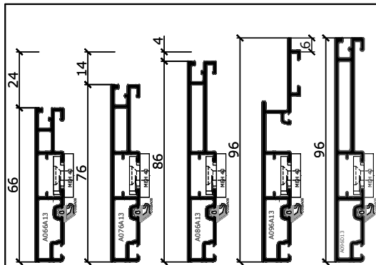
Ausführungsvarianten Blendrahmenprofil
