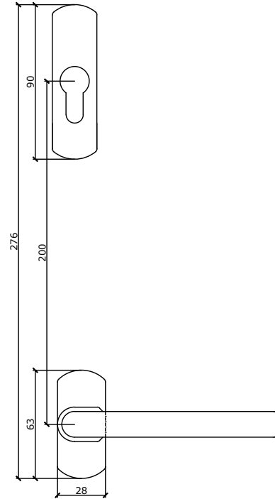
abschliessbarem Getriebe
