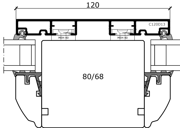
Rahmensprosse
