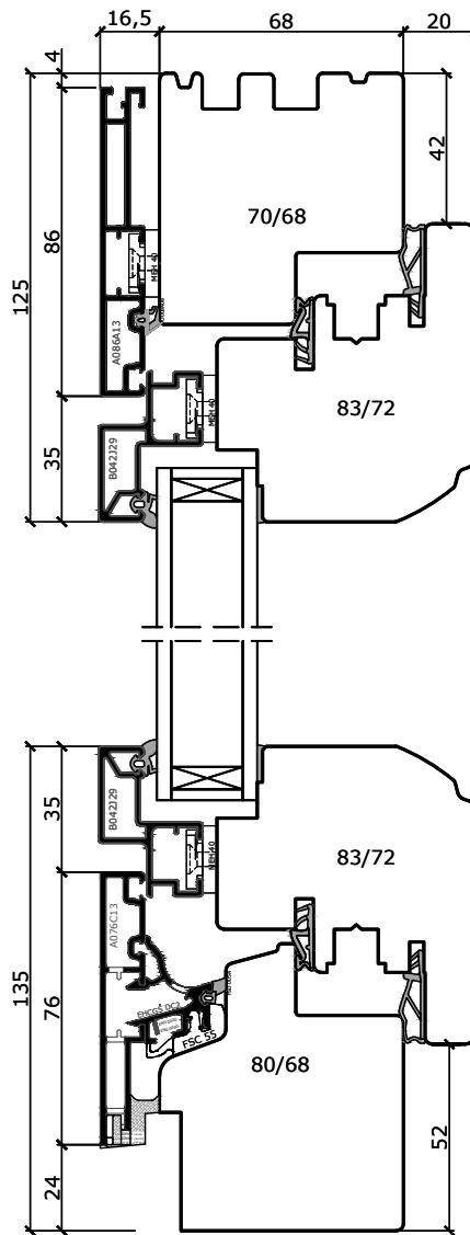
Ausführungsvarianten Innenprofil
