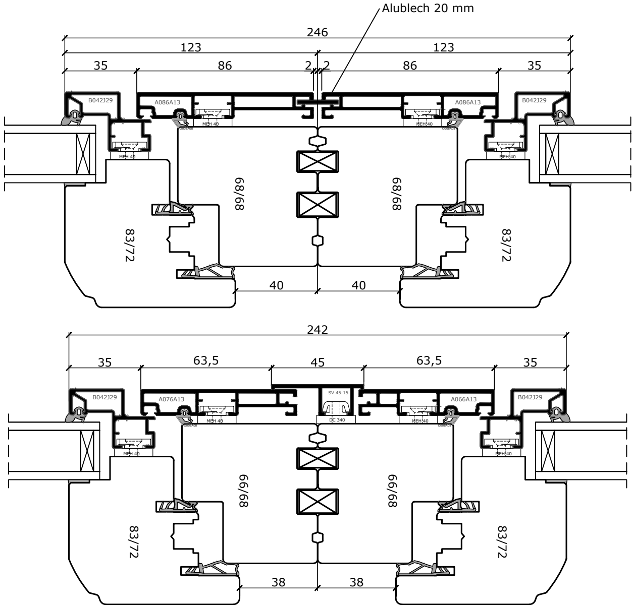
Verbreiterungsprofile
