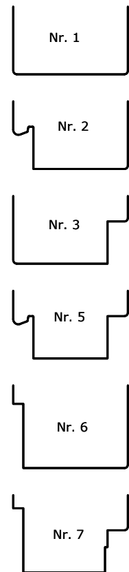
Ausführungsvarianten Fensterbankanschluss
