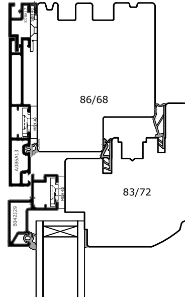
Rahmenverbreiterung mit Verbreiterungsprofil J028A20 Immer 6 m Stangen kalkulieren und Holzbreite über 80mm kalkulieren
