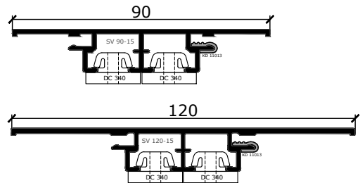
Verbreiterungsprofile mit Blechaufnahme mit Dichtung KD 11013:
