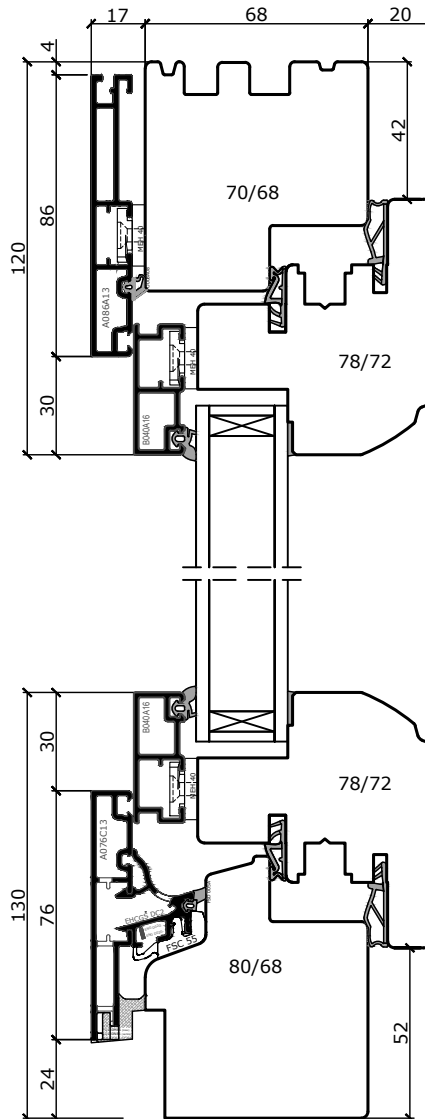
Ausführungsvarianten Innenprofil
