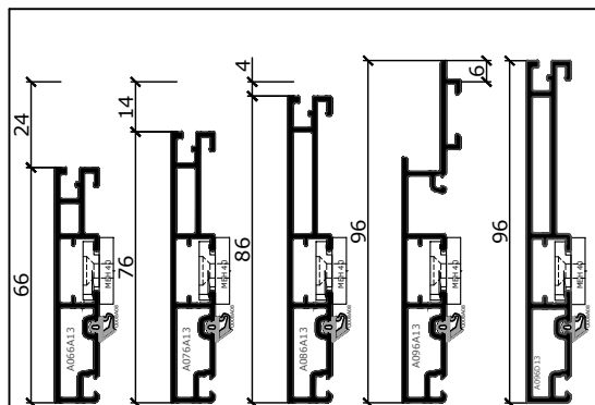
Ausführungsvarianten Blendrahmenprofil
