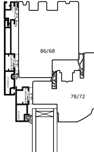
Rahmenverbreiterung mit Verbreiterungsprofil J028A20 Immer 6 m Stangen kalkulieren und Holzbreite über 80mm kalkulieren
