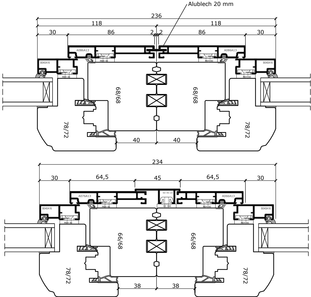
Verbreiterungsprofile
