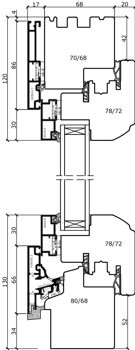
System IV68 Glasstärken von 28 bis 48 mm
