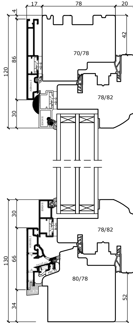
System IV78 Glasstärken von 38 bis 54 mm
