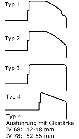
Ausführungsvarianten Innenprofil
