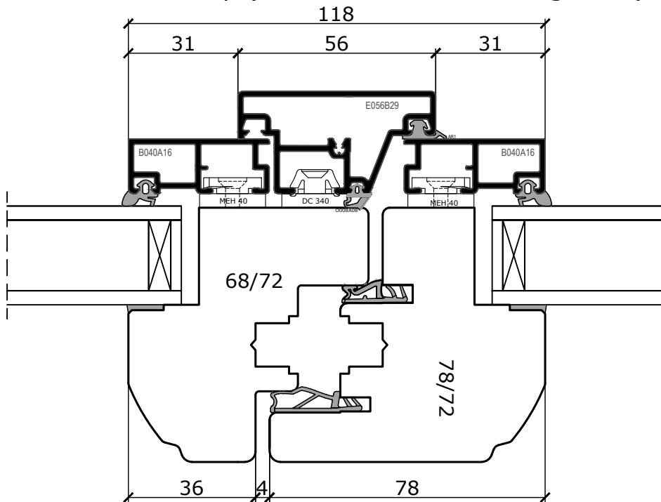
Schmäler Stulp (nicht bei Balkontüre möglich!!!)
