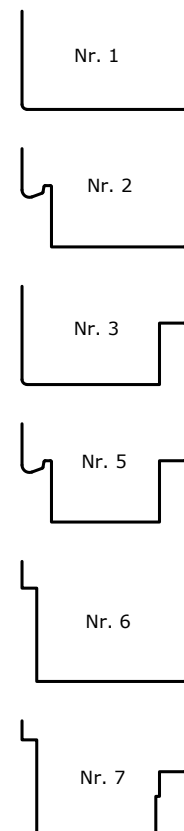
Ausführungsvarianten Fensterbankanschluss
