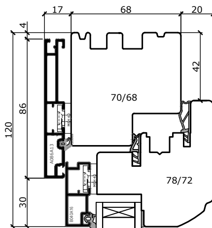
Ausführungsvarianten Innenprofil
