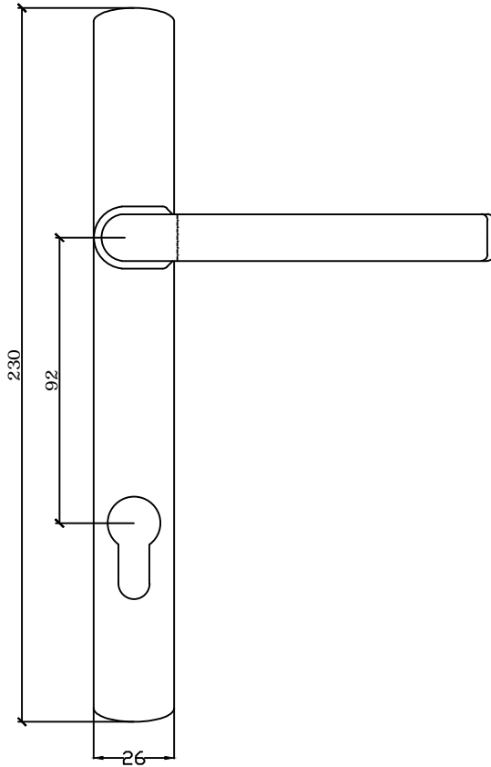
BTV (Balkontürverschluss)
