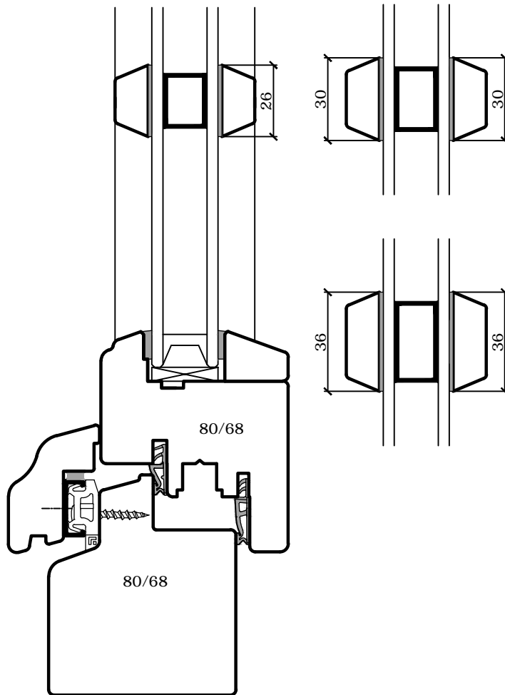
Standard Wiener Sprosse
