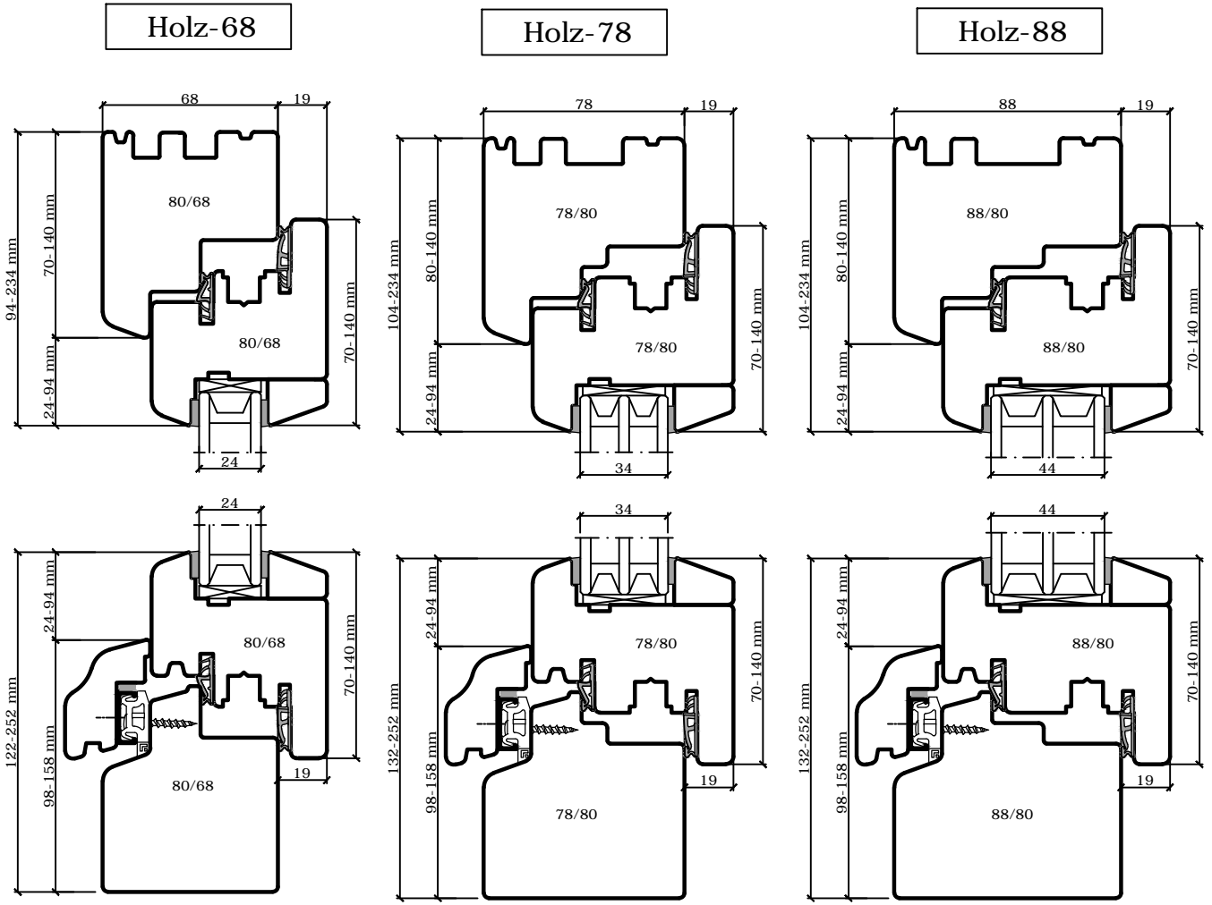
System IV68 Glasstärken von 24 bis 30 mm
